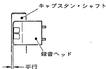
図15 録音ヘッドのあおり調整
