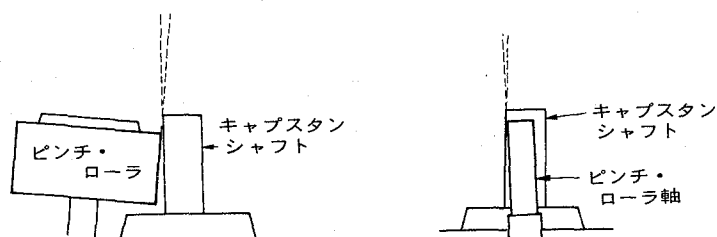
図11 A視図(平行でない例)
