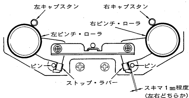
図3 ピンチ・ローラ圧着調整
